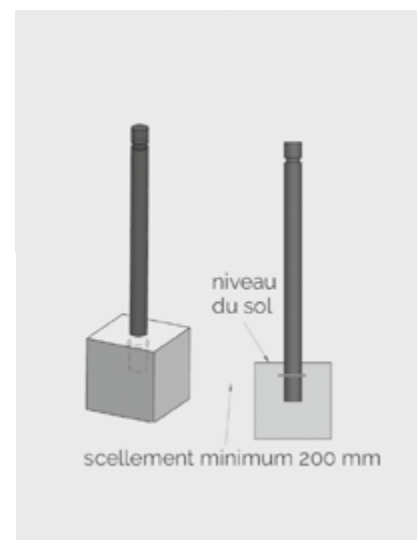
Potelet avec fer à béton
